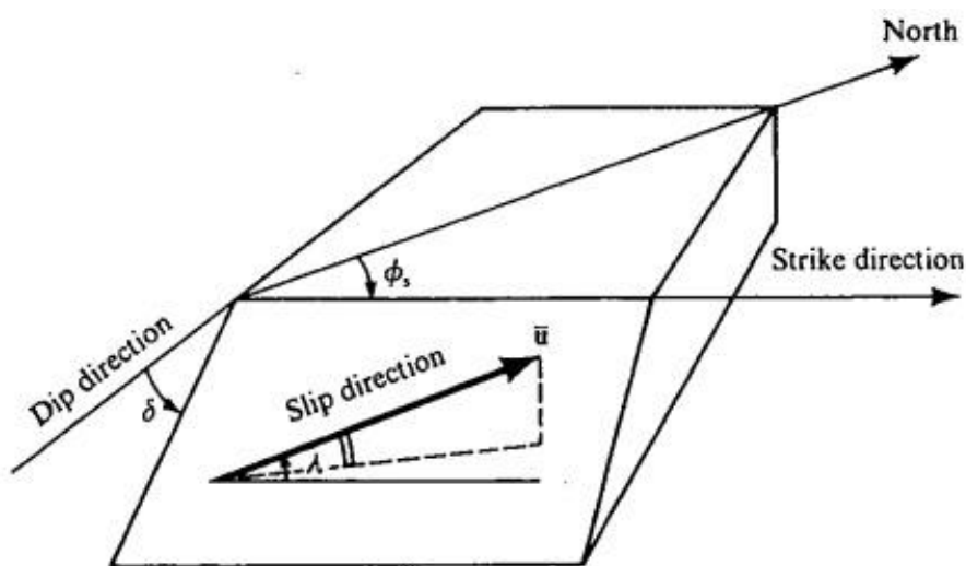
Рисунок 4.5- Направления простираания, падения и угла наклона [95]
