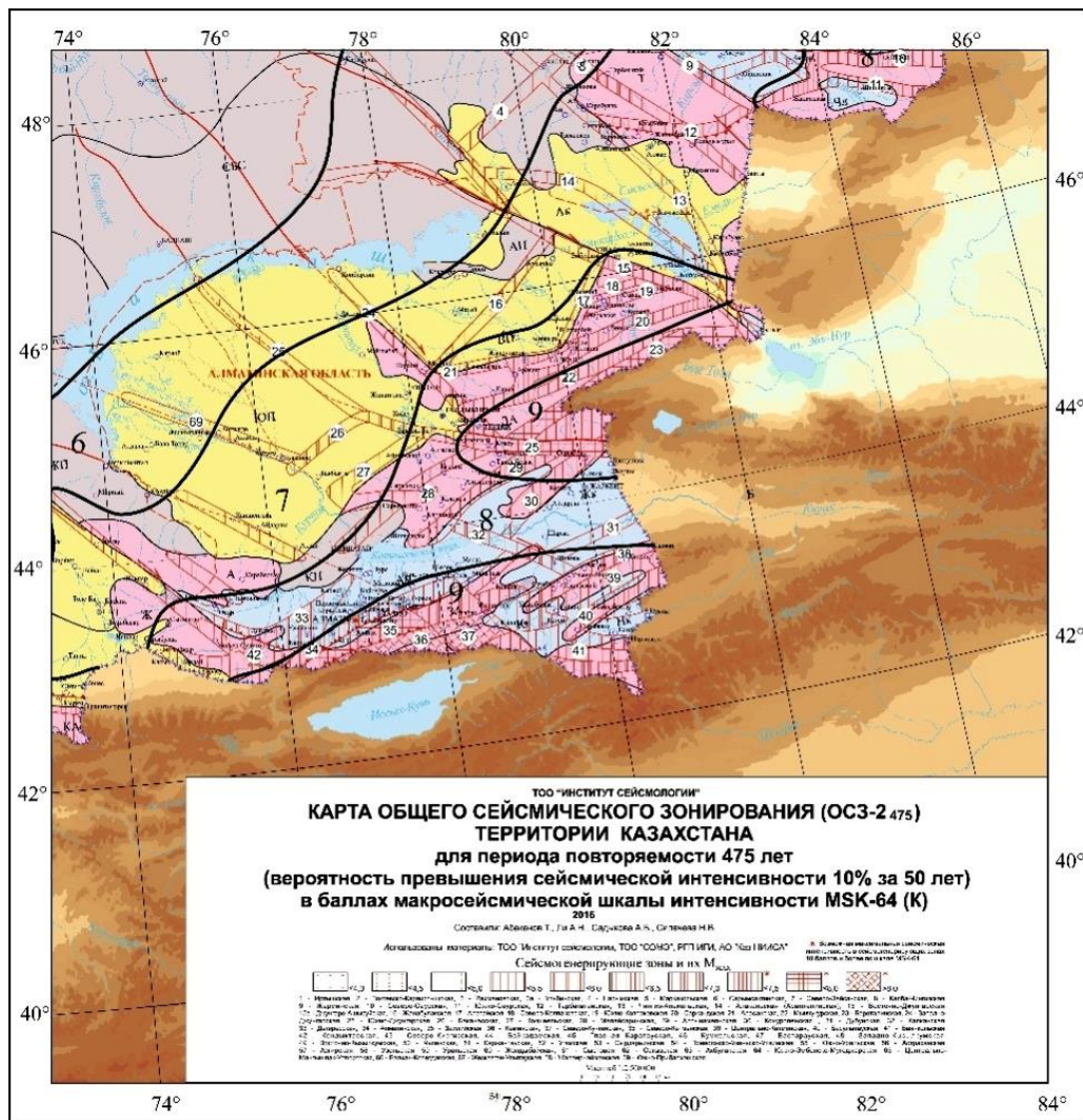
Рисунок 4.14-Карта общего сейсмического зонирования территории Северо-Тянь-Шаньского региона в баллах макросейсмической шкалы интенсивности MSK-64 (K)
