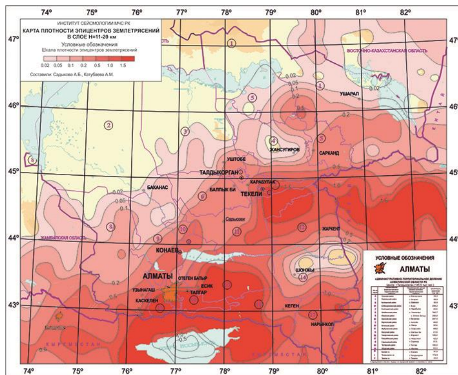
Рисунок 5.6 – Карта плотности эпицентров землетрясений с глубинами H=11-20 км
