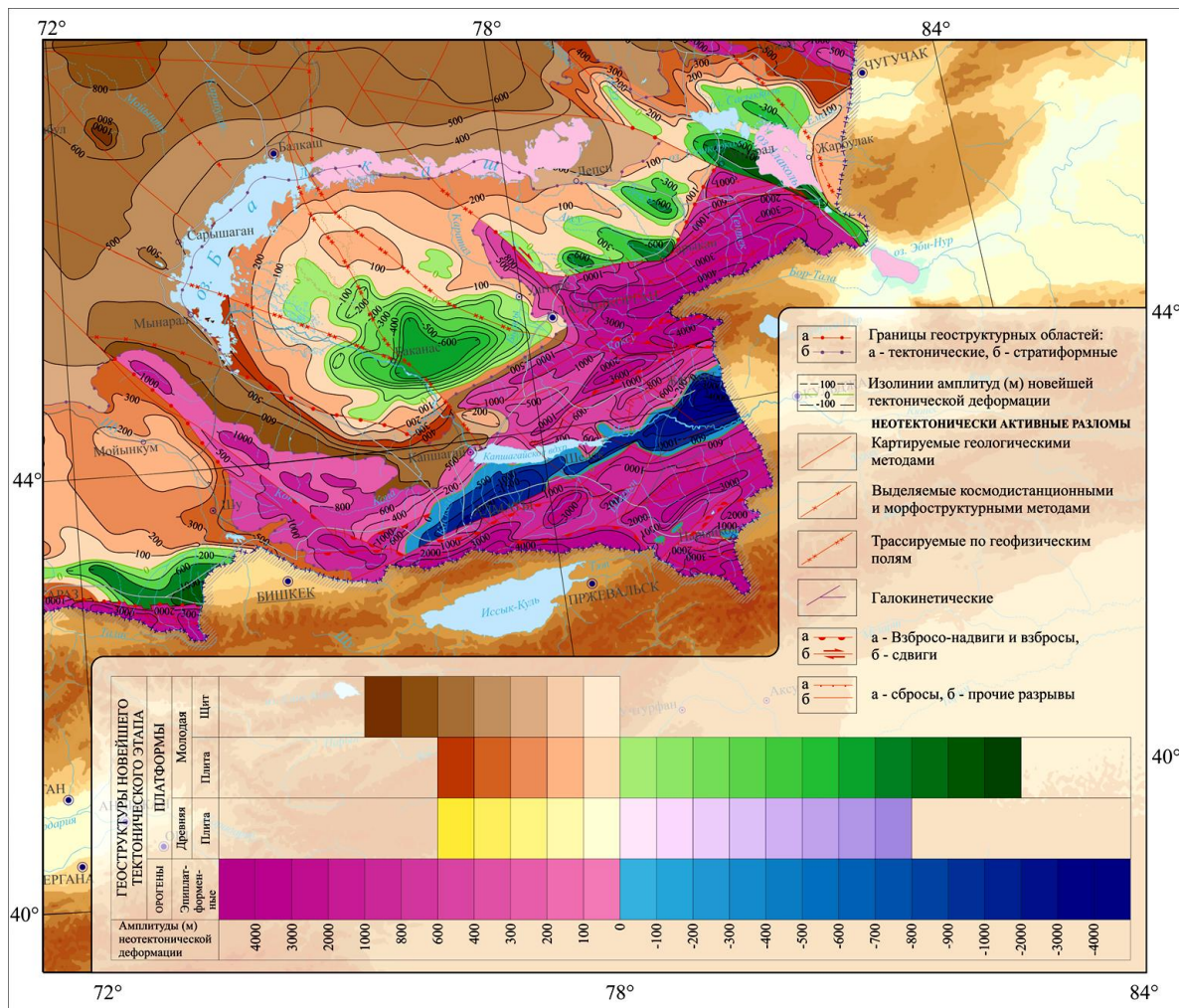
Рисунок 2.2 - Карта новейшей тектоники Жонгаро-Северо-Тянь-Шаньского региона [29]
