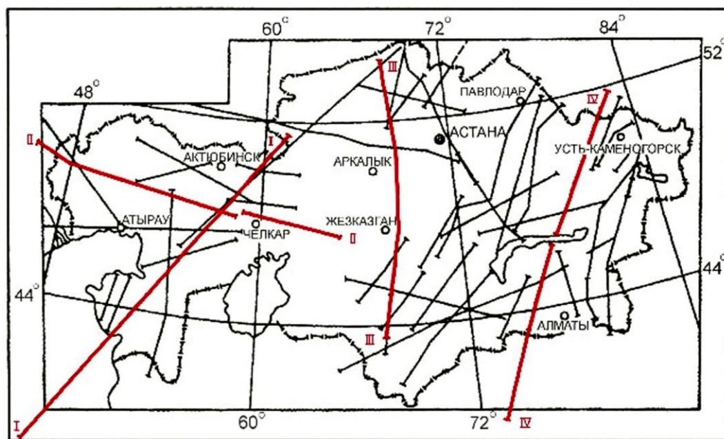
I-I – Баку-Кустанай, II-II – Волгоград-Челкар-Тургайский, III-III – Каратау-Николаевка, IV-IV – Памир-Сарыташ-Саякский
