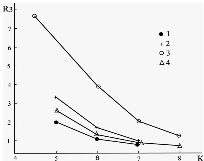
Рисунок 6.15- Зависимость параметра R_3=N_{\text{н}}/N_{\text{дн}} (отношение количества событий в дневные и ночные часы) от энергетического класса землетрясений для исследуемых зон: 1 – Северо-Тянь-Шанская; 2 – Жонгарская; 3 – Халыктауская; 4 – Кетменьская
