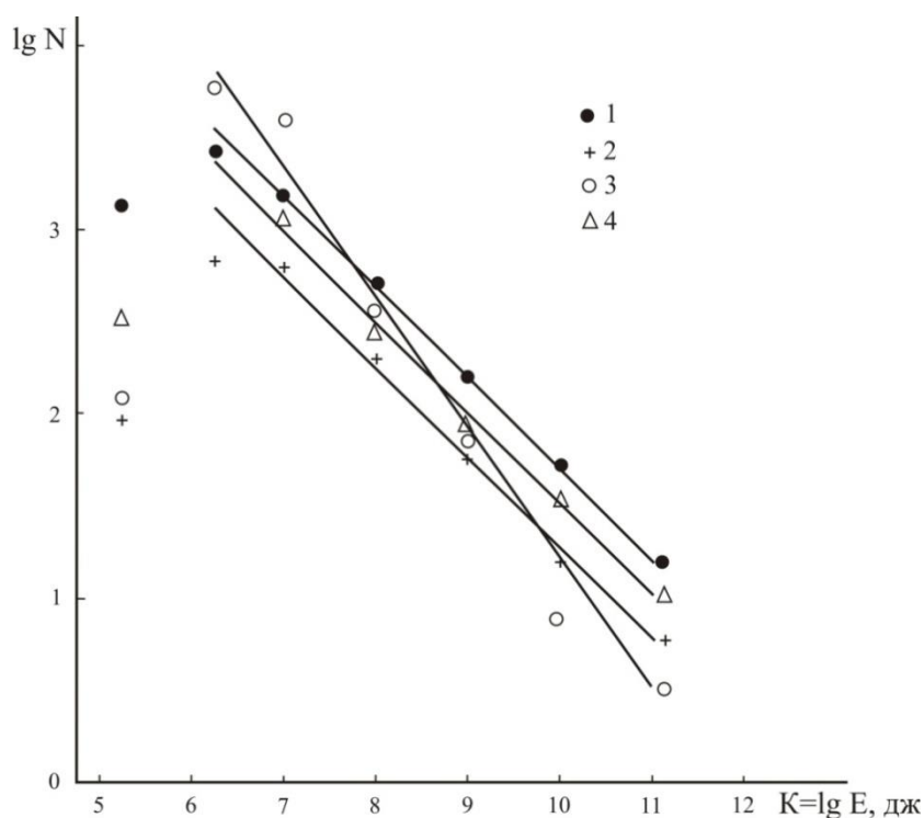
Рисунок 6.9 - Графики повторяемости землетрясений за период 2004-2010 гг. для четырех исследуемых зон: 1 – Северо-Тянь-Шаньская; 2 – Жонгарская; 3 – Халыктауская; 4 – Кетменьская
