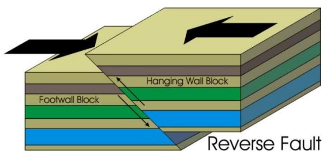
Рисунок 4.3 - Типичный взброс [94]
