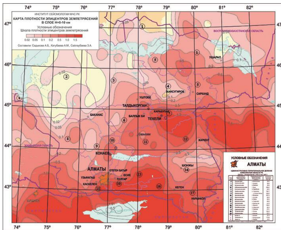
Рисунок 5.5 – Карта плотности эпицентров землетрясений в близповерхностном слое H=0-10 км
