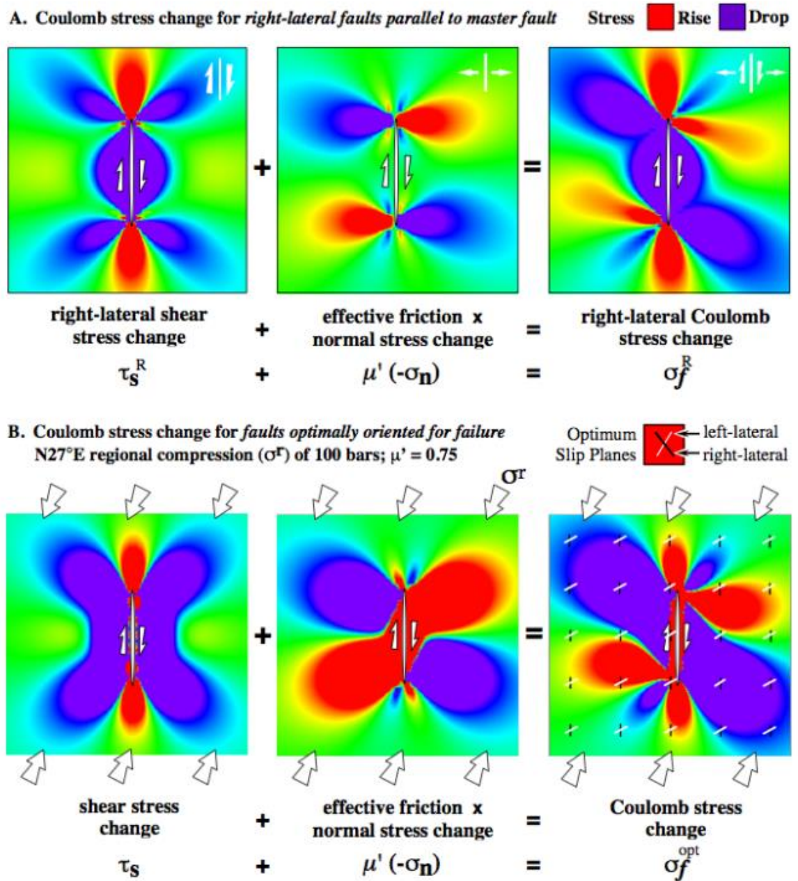
Рисунок 4.1. Иллюстрация изменения кулоновского напряжения [93]
