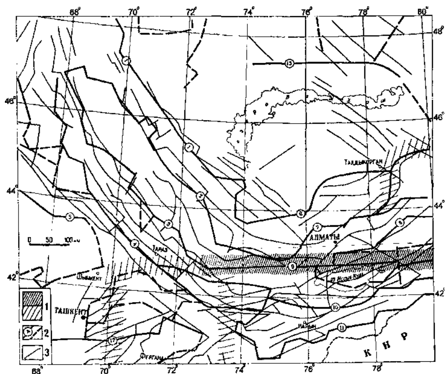
1 – сквозькоровые флексурно-разломные зоны, выделенные по высоким горизонтальным градиентам силы тяжести первого (а) и второго (б) порядков; 2 – разломы в сиалическом цоколе гранито-гнейсового слоя до глубины 15-20 км первого (а) и второго (б) порядков (цифры в кружках): 1 – Жалаир-Найманский, 2 – Чуйский, 3 – Жезказган-Таласский, 4 – Каратау-Ферганский, 5 – Южно-Каратауский, 6 – Кокшаальский, 7 – Алтынэмельский, 8 – Северо-Кетменский, 9 – Северо-Тянь-Шаньский, 10 – линия Николаева, 11 – Атбаши-Иныльчекский, 12 – Северо-Ферганский, 13 – Бектаутинский;
