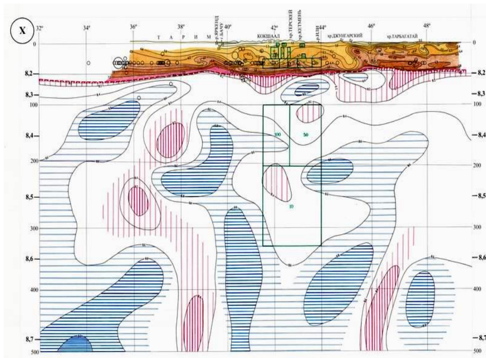
I – геотраверс Северо-Тяньшаньский (41.25N, 69.167E; 44.083N, 90.00E). X – геотраверс Восточный (32.00N, 77.41E; 45.216N, 80.0678E; 49.00N, 83.667E).
